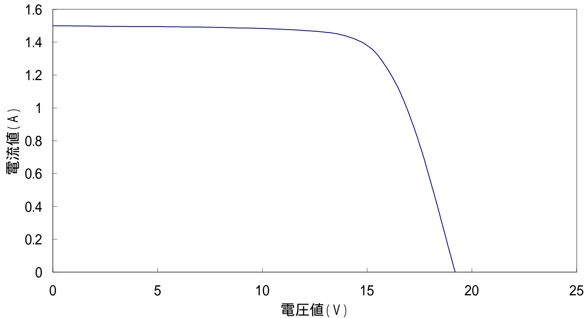
KGX20 出力特性図 @1000W/m 2 AM1.5 25
